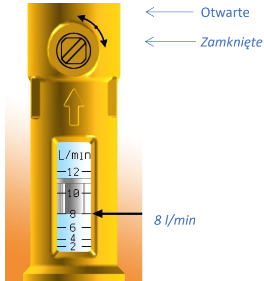
Rys 8. Korpus przepływomierza liniowego PRAWTECH serii A: 2-12 l/min
