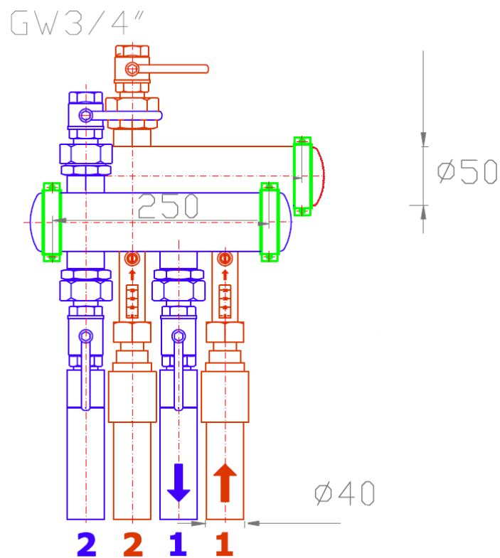
Rys 3. Rozdzielacz szafki Terra BOX z rotametrami 2 sekcje zewnętrzny
