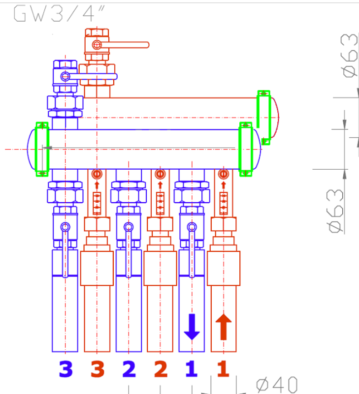
Rys 4. Rozdzielacz szafki Terra BOX z rotametrami 3 sekcje zewnętrzny
